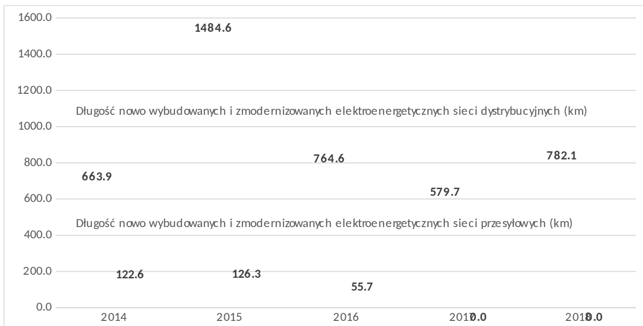
Wykres 10. Długość nowo wybudowanych i zmodernizowanych elektroenergetycznych sieci dystrybucyjnych oraz długość nowo wybudowanych i zmodernizowanych elektroenergetycznych sieci przesyłowych w latach 2014-2018
